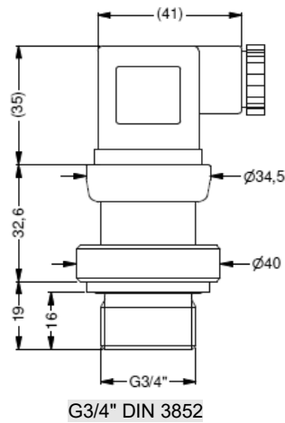
G3/4" DIN 3852
